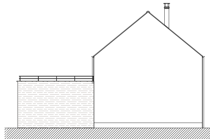
FACADE OUEST
